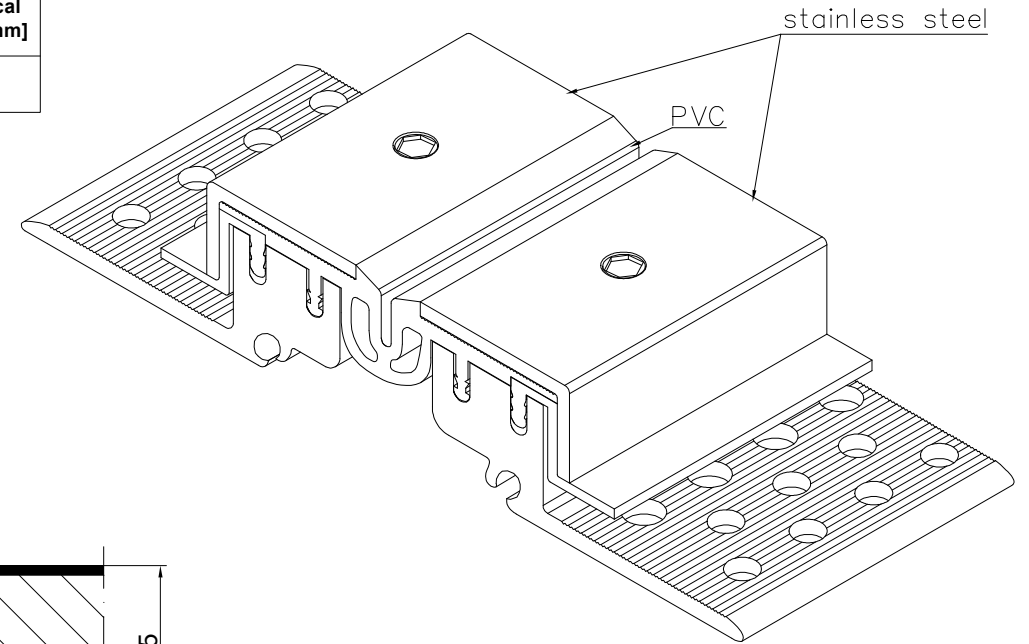
CONECTO GA 43.10.35 S VIEW
