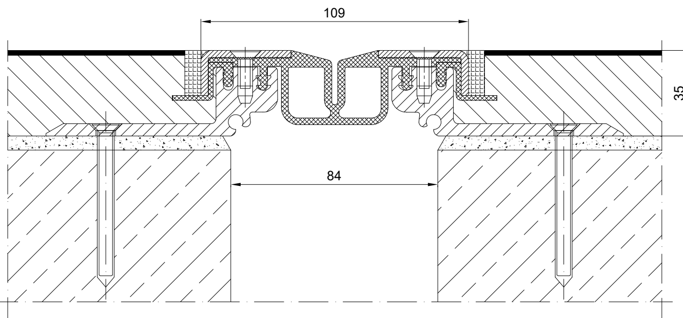
CONECTO GA 63.30.35 S SECTION
